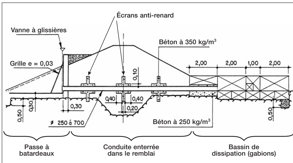
Vue en coupe d'un organe de vidange constitué d'une conduite enterrée sous le remblai et commandée à l'amont par une passe à batardeaux [3]
